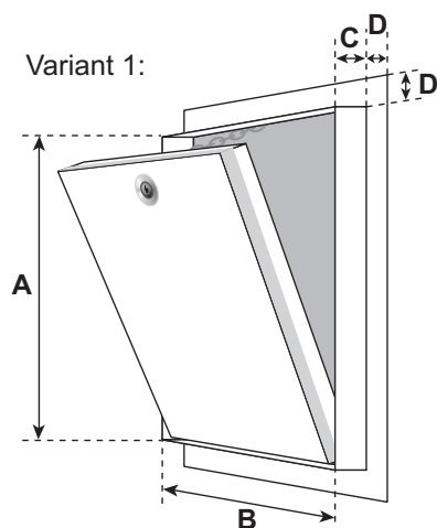
Beszerelés hagyományos falba
